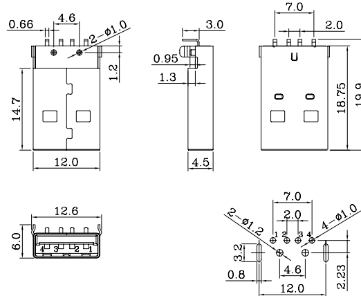
PCB LAYOUT 线路板布局图
