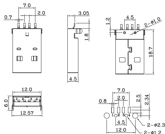
PCB LAYOUT 线路板布局图
