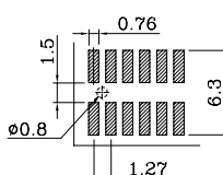
PCB LAYOUT 线路板布局图
