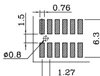
PCB LAYOUT 线路板布局图
