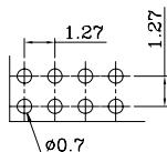
PCB LAYOUT 线路板布局图
