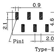
PCB Layout 线路板布局图
