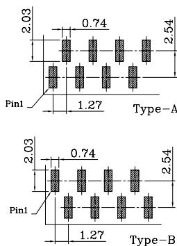
PCB LAYOUT 线路板布局图
