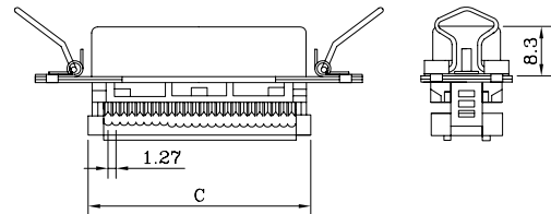
57F-40 系列
