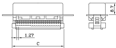
57F-30 系列
