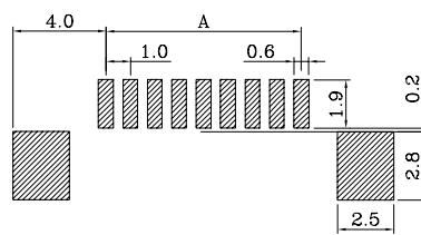
PCB LAYOUT 线路板布局图
